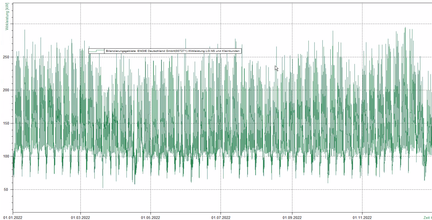
Bild 1: Lastverlauf MS als viertelstündliche Leistungsmessung
