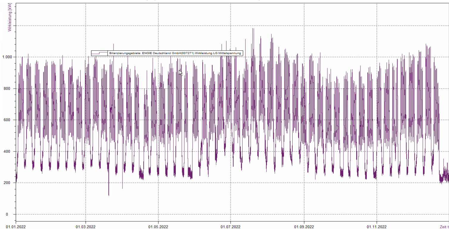
Bild 1: Lastverlauf MS als viertelstündliche Leistungsmessung
